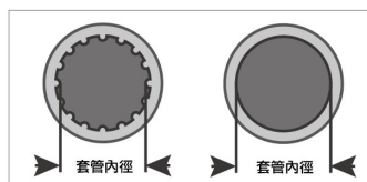
市售 PVC 套管 (內緣有爪、無爪皆適用)
